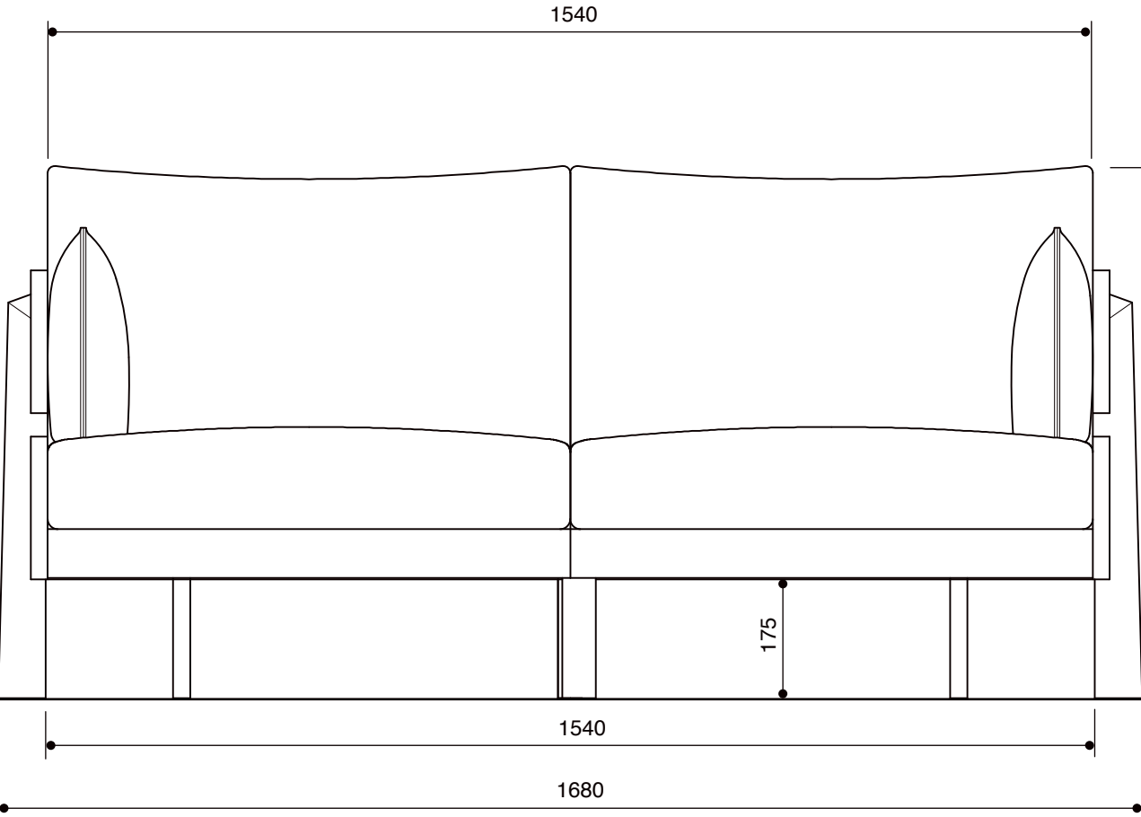
【正面】
